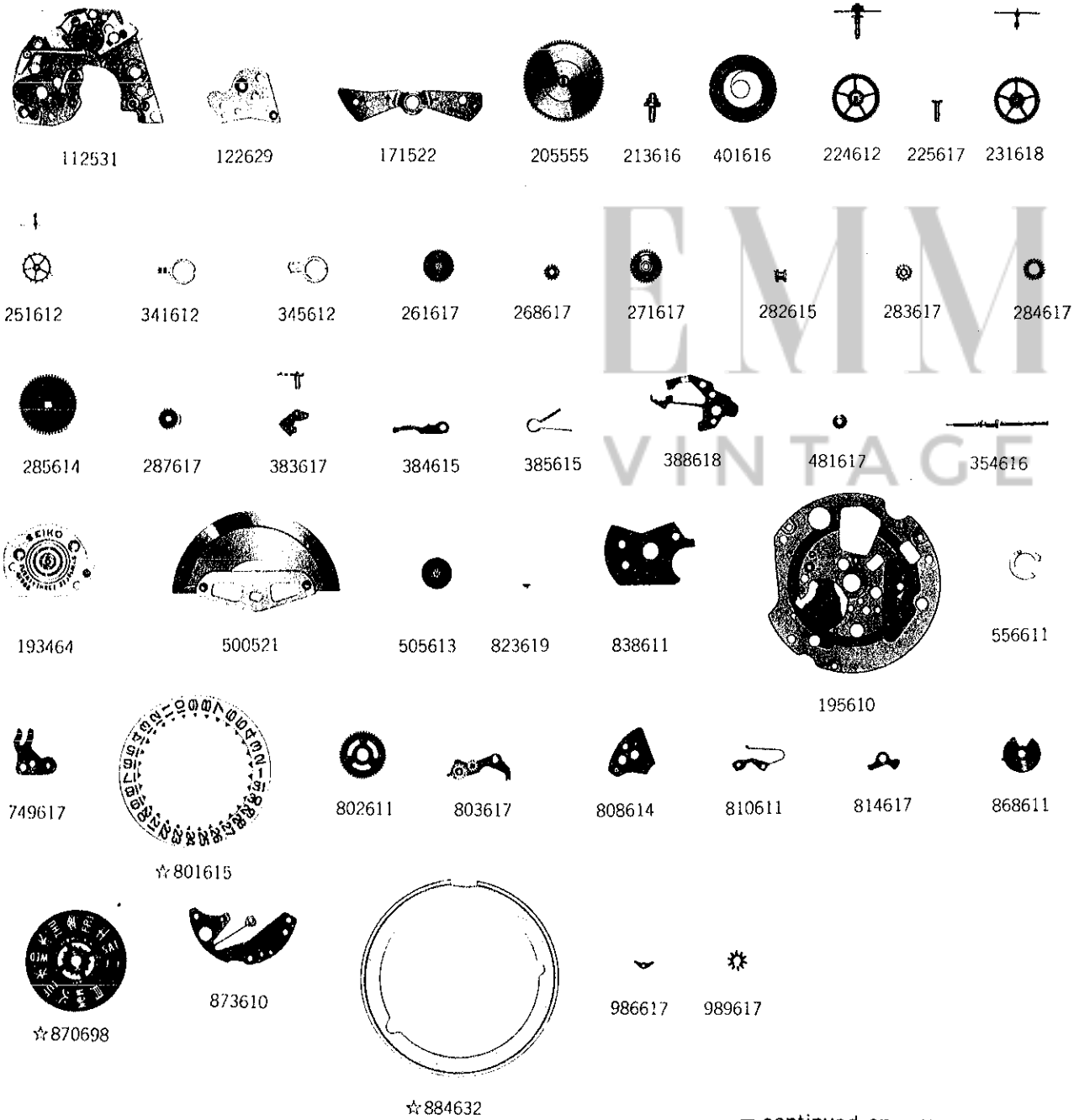
Cal. 6138B
