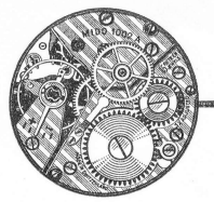
10 ½''' - 1002 A seconde au centre (SC) center second (CS)
