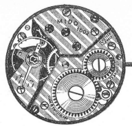
10 ½''' - 1002 seconde habituelle small second
