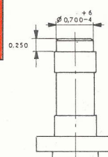
Chaussée Cannon pinion Minutenrohr 分輪
