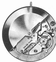
13 1/2''' cal. 1582 calendrier à bague
