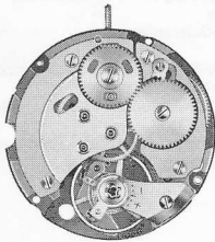
Cal. 2084
