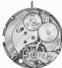
Cal. 2184
